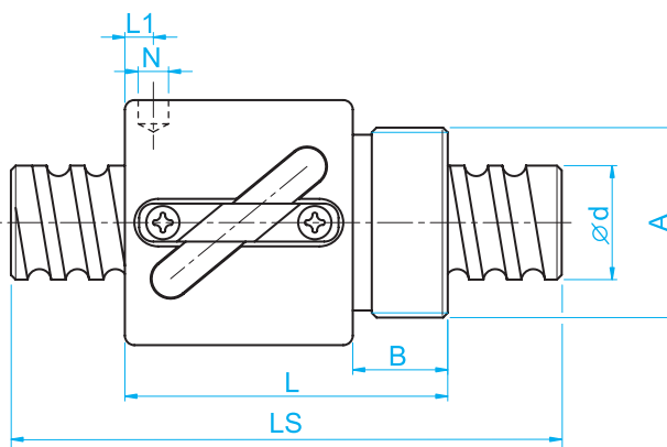
d \leq 14 (External circulation type) 外循環
