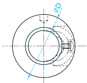
d \leq 14 (External circulation type) 外循環
