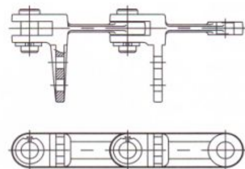
Case Chain [ 特殊链条 ]
