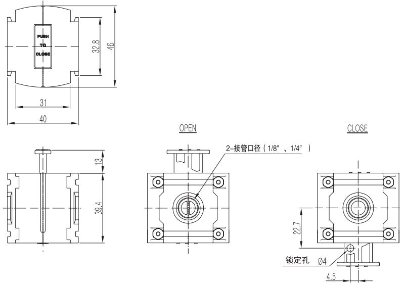
PLV2尺寸图
