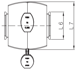
PLV3、4、5尺寸图
